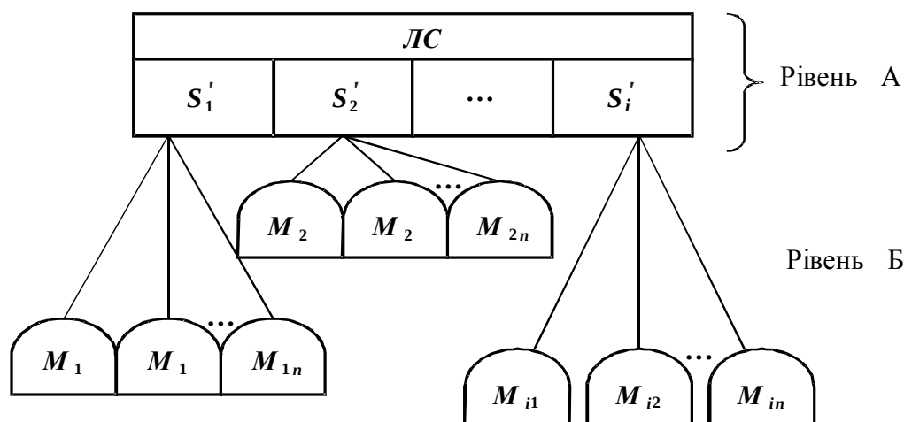
Рис. 2.10. Схема радіальної структури системи*
